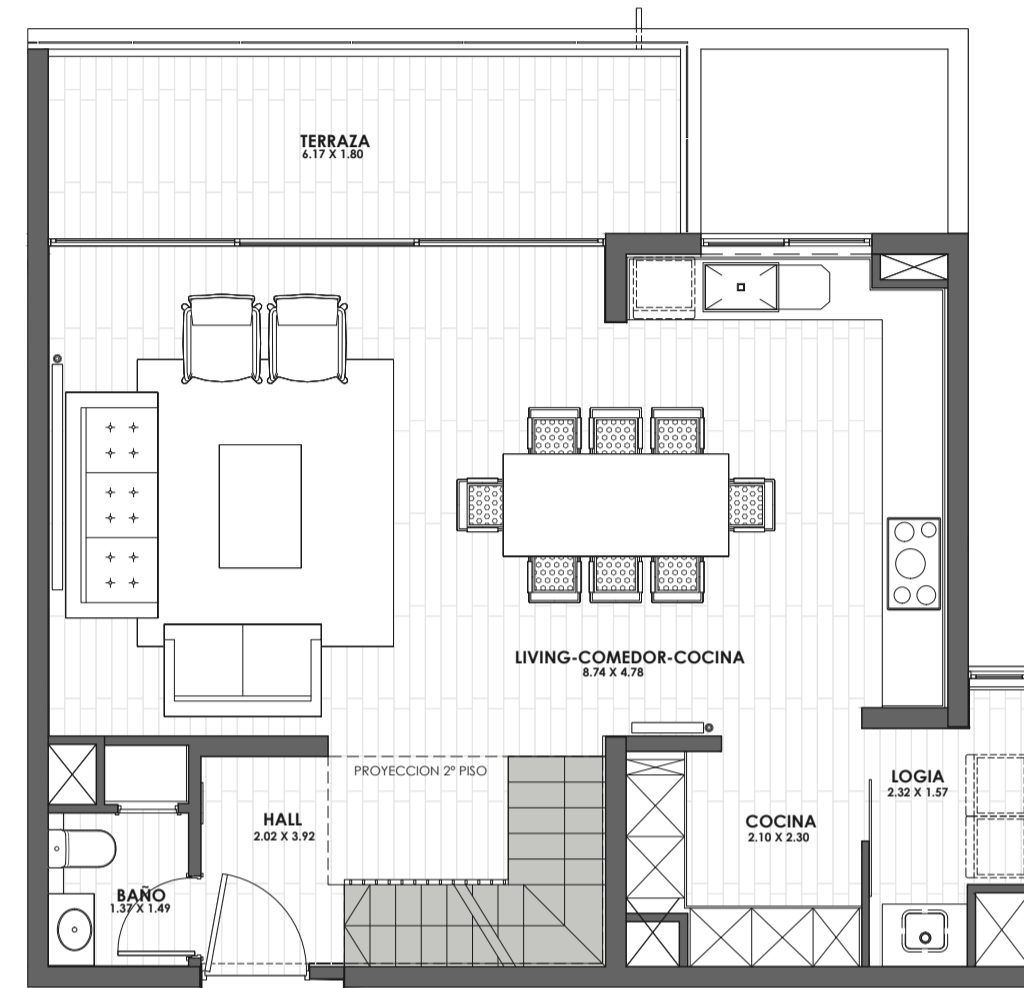
NIVEL ACCESO (PISO 7°)
