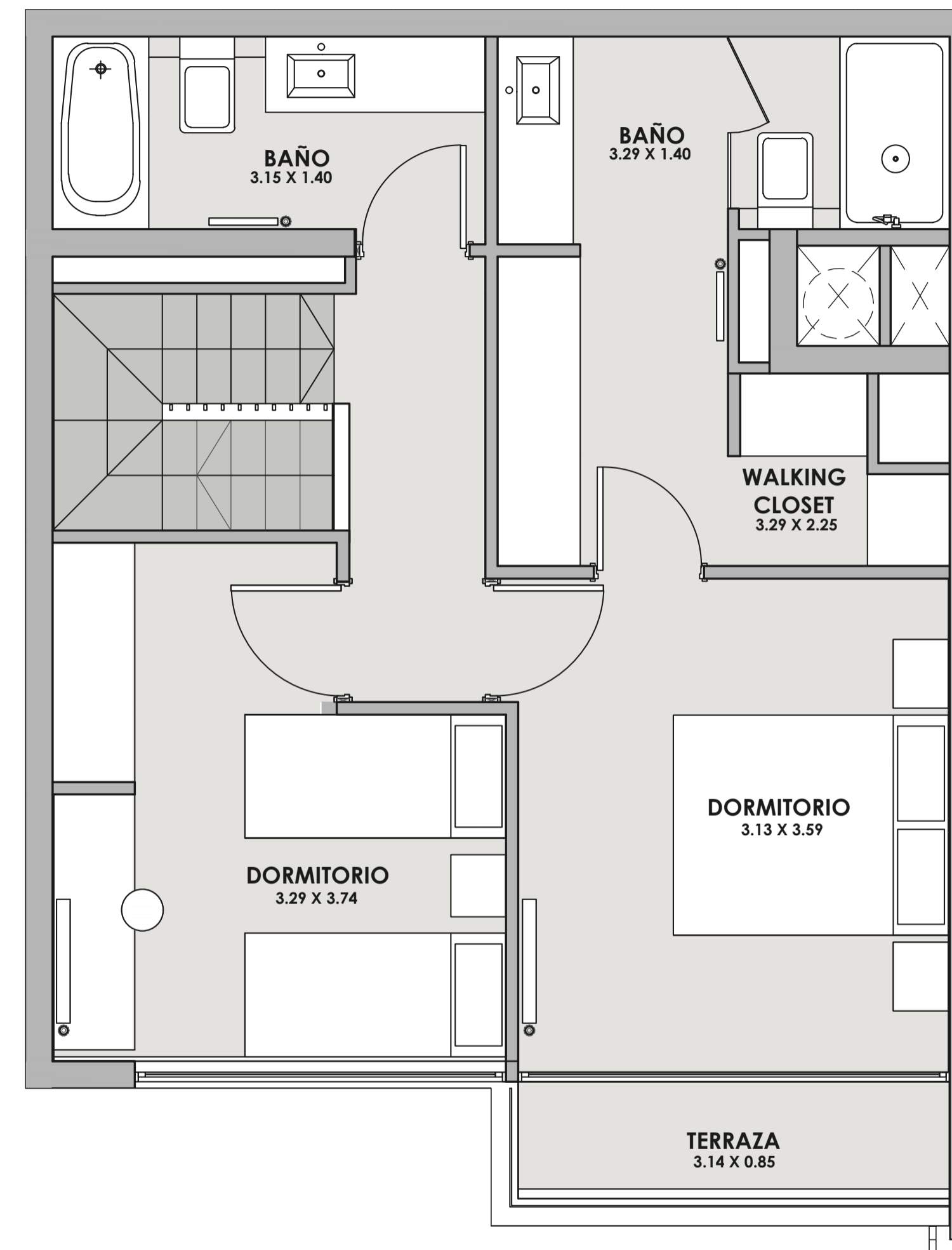
NIVELES SUPERIORES (PISO 3º Y 5º)
