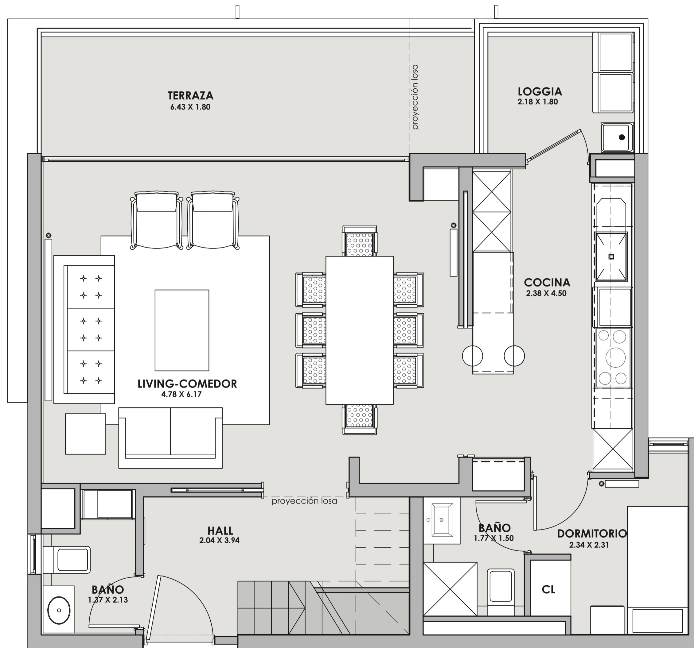
NIVELES ACCESO (PISOS 2° Y 4°)
