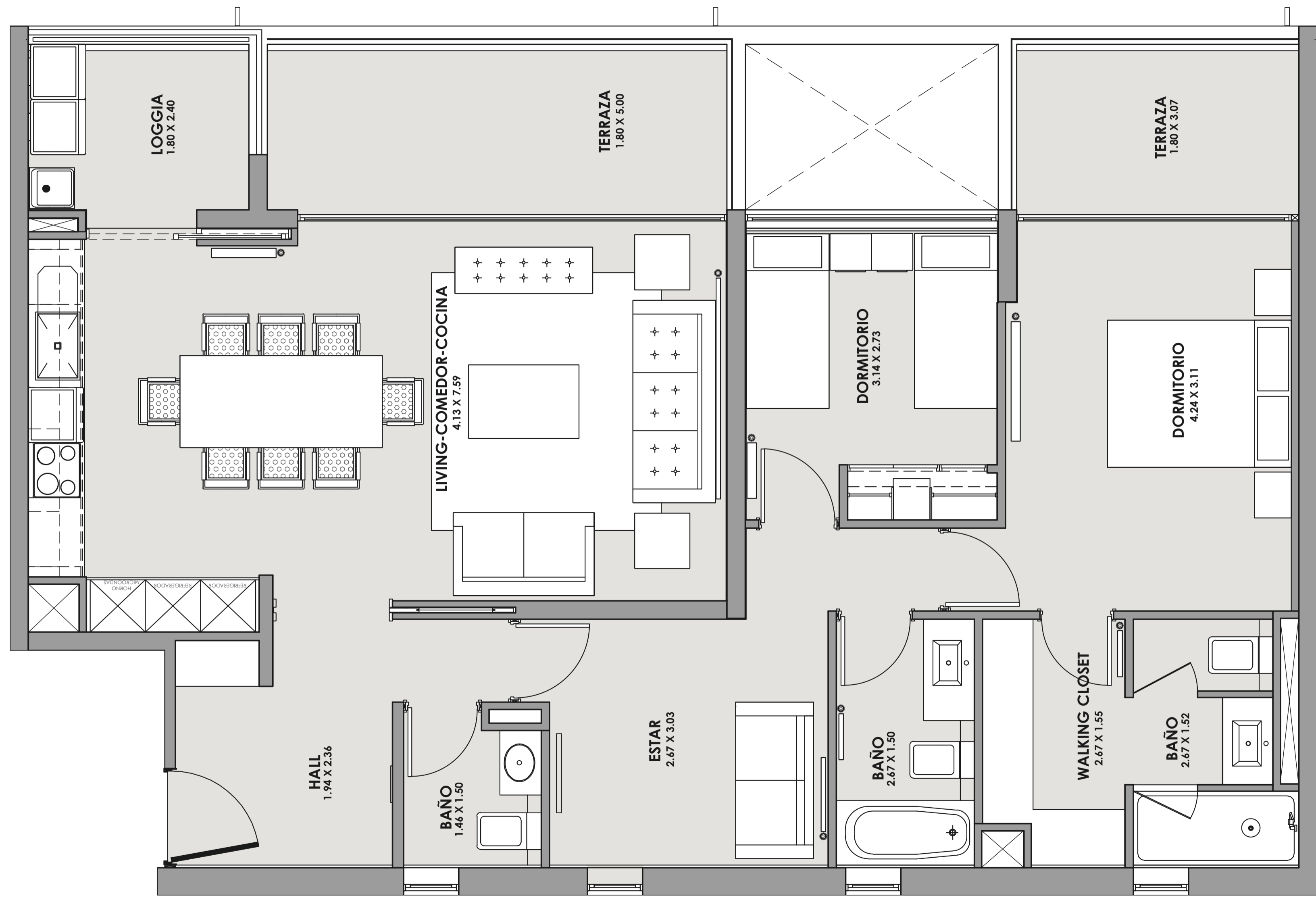
DEPARTAMENTO 203 - 303 - 403 - 503 - 603
